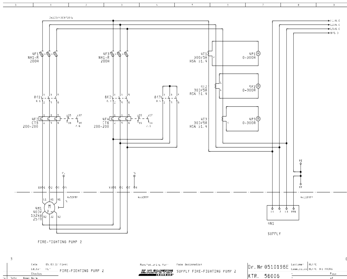
Hình 1.3: Sơ đồ động lực
