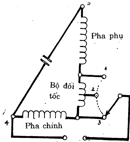
Sơ đồ nguyên lý mạch đổi tốc hình T
