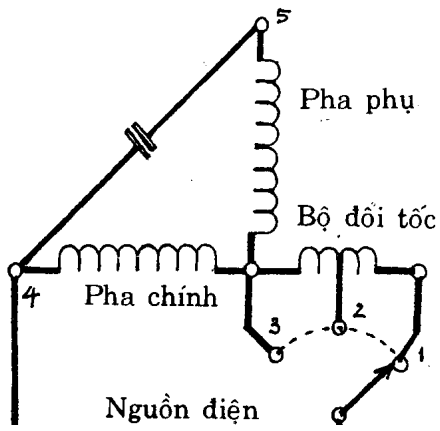
Sơ đồ nguyên lý mạch đổi tốc hình T
