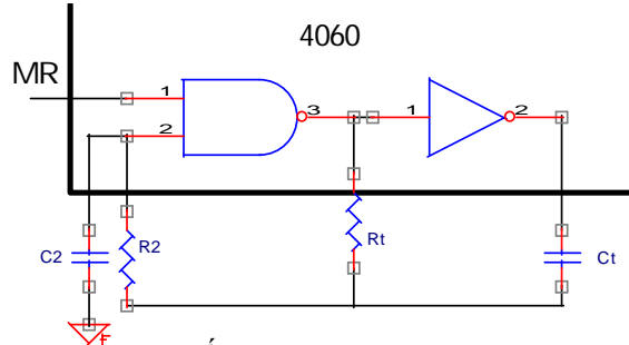
Mạch kết hợp RC bên ngoài IC 4060
