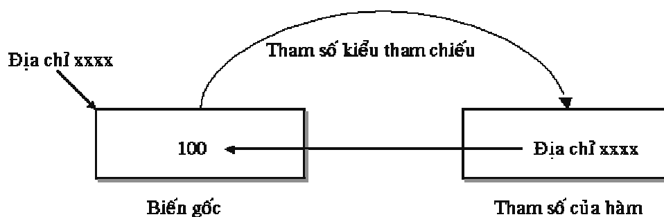
Hình 2.14: Một tham số kiểu tham chiếu nhận một tham chiếu tới một biến được chuyển cho tham số của hàm.
