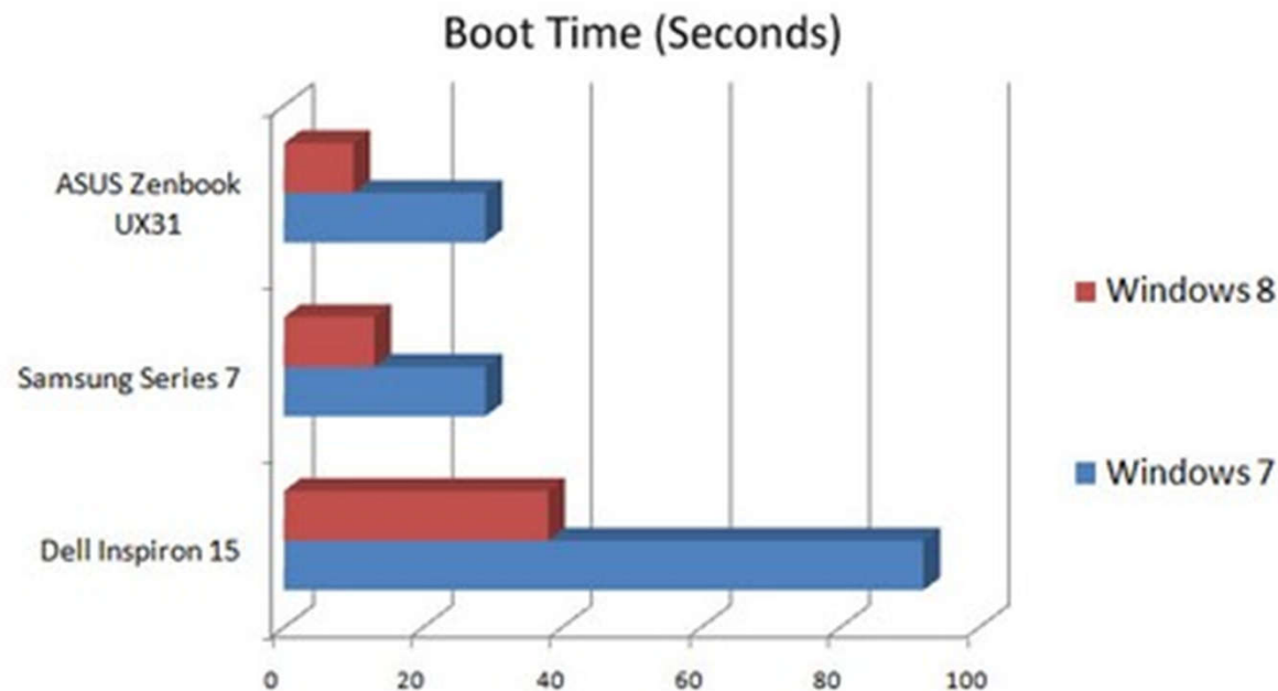
Hình 1 :Biểu đồ so sánh tốc độ khởi động của Windows 7 và Windows 8 trên cùng 1 máy tính (ngắn hơn là nhanh hơn)
